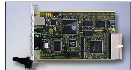
DF PROFI II CPCI
